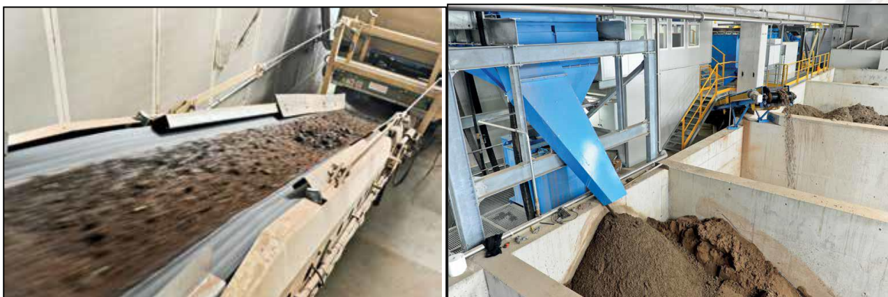
Figura 4: Impianto di trattamento terre - Soil washing
