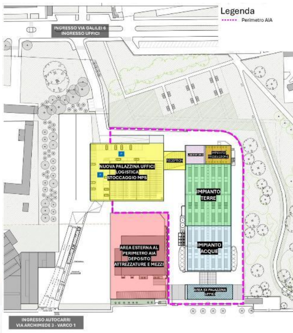
Figura 9: Planimetria Sito SEMP
